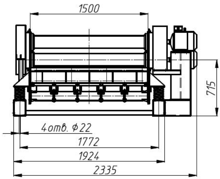
Вид А
